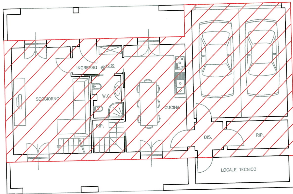
PLANIMETRIA PIANO TERRA 110 MQ SUL
