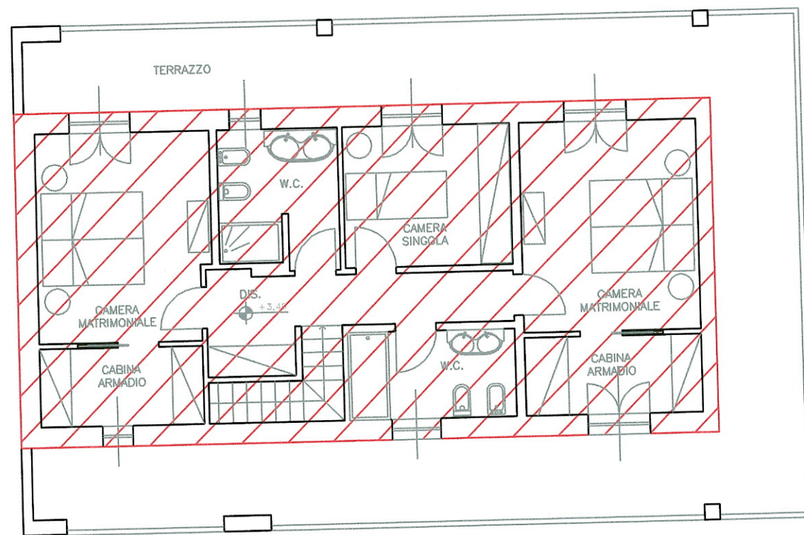
PLANIMETRIA PIANO PRIMO 90 MQ SUL
